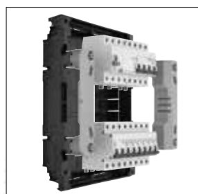
5 AJUSTE DEL CHASIS El chasis permite la nivelación para compensar las imperfecciones en la instalación de la caja
